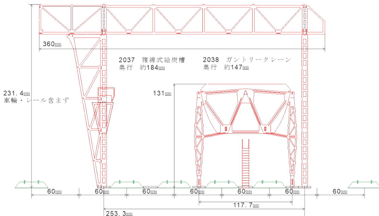
組立例 車両、線路並びに一部土台板は撮影用。 キットには含まず。写真は試作品です。
